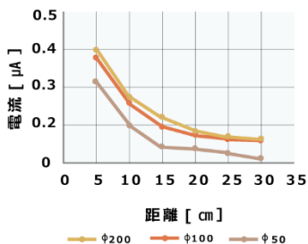
電流測定試験
