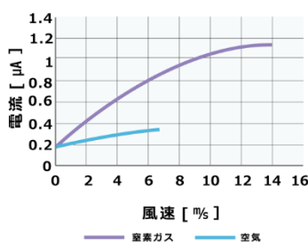
空気と窒素の除電効果試験
