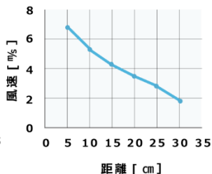
射程距離試験
