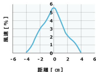
風の広角試験 (10cmの時)
