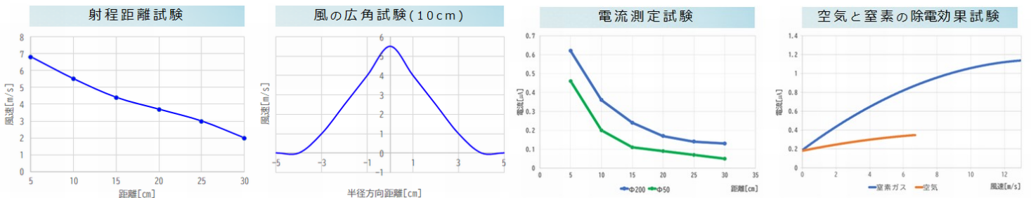
イオナイザーガン主要データ
